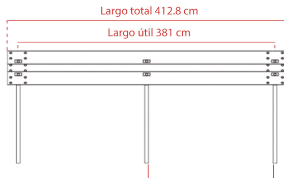
Pruebas impactadas y superadas Nivel de contención NC-4 (MASH)
